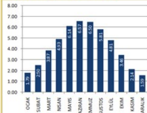
TÜRKİYE Global Radyasyon Değerleri (KWh/m².gün)
