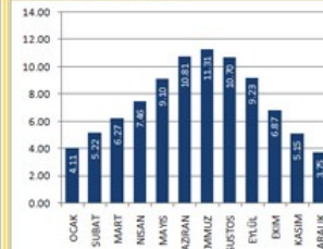
TÜRKİYE Güneşlenme Süreleri (Saat)
