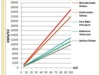
TÜRKİYE PV Tipi Alan Üretilebilecek Enerji (KWp.Yıl)
