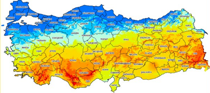
TÜRKİYE Global Radyasyon Değerleri (KWh/m².gün)
